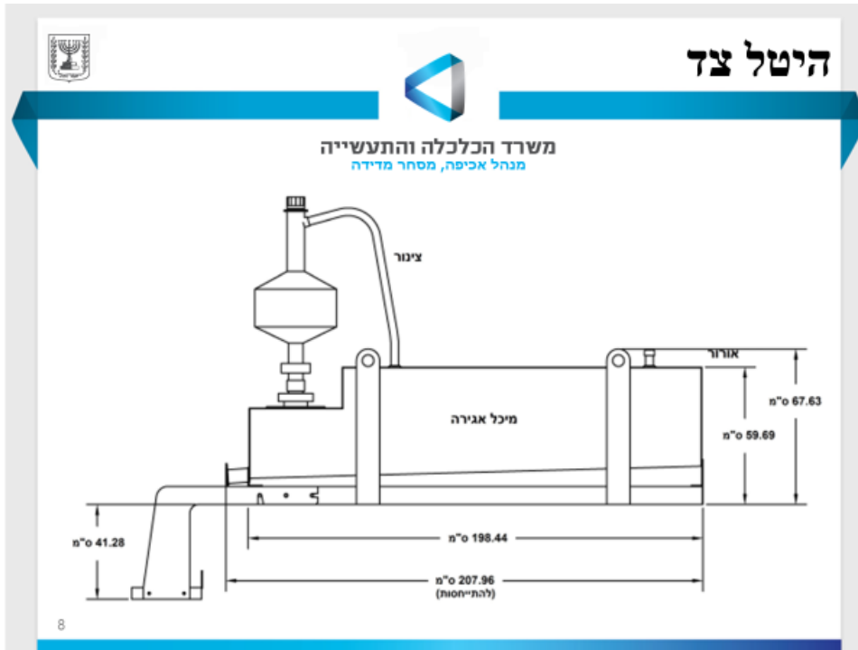
איור 3 : מערכת כיוול ייעודית היטל צד
