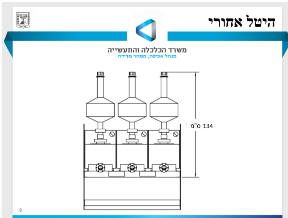
איור 4 : מערכת כיוול ייעודית היטל אחורי
